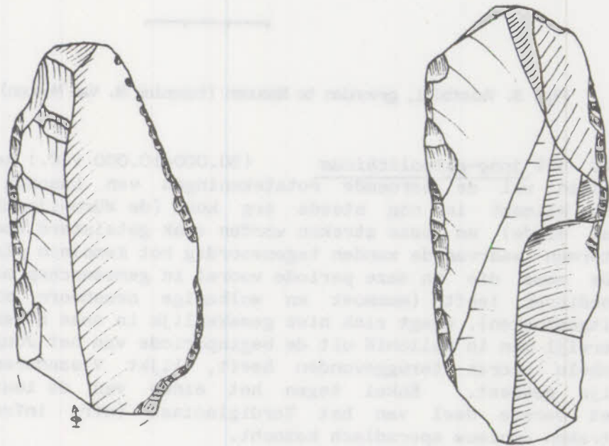
Fig. 2. Boordschrabbers gevonden te Opglabbeek. Links : Ruiterskuilen. Rechts : Turfven (tekening naar Creemers, 1985).
